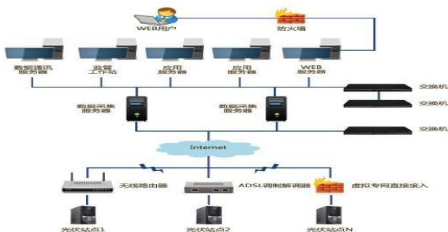
图5.8-1 监控和通讯原理图
